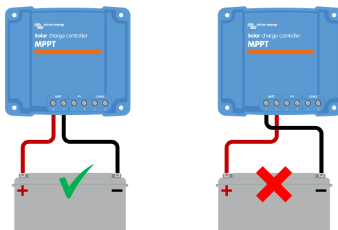
Beispiele für richtige und falsche (vertauschte) Batteriepolartät.
